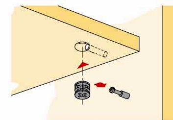
Рис.2 Схема сборки стяжки эксцентриковой
