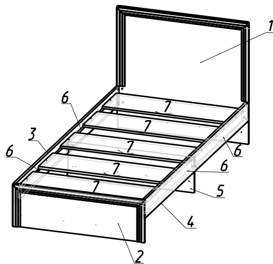
Рис.1 Схема сборки
